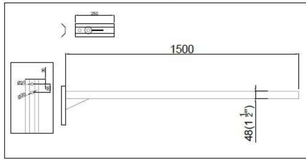
DETALLE A
